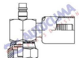
ŻEŃSKA - O.RING - 90° - PORT R134a
