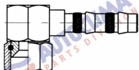
FRIGO - 90° - FLARA - ŻEŃSKA
