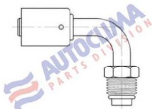
MĘSKA - O.RING - 90°
