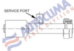
ŻEŃSKA - 180° - ROTOLOCK PORT R134a
