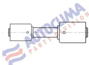
ZŁĄCZKA REDUKCYJNA
