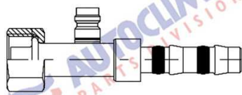
FRIGO - 180° - O.RING - ŻEŃSKA PORT R134a
