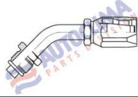
KOŃCÓWKA BUS - 45° MĘSKA - O.RING
