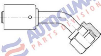
KOŃCÓWKA ŻEŃSKA - O.RING - 45°
