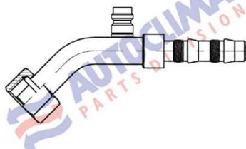
FRIGO - 45° - O.RING - ŻEŃSKA PORT R134a
