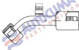
ŻEŃSKA - O.RING - 45° - PORT R134a
