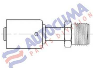
MĘSKA - O.RING WEWN.- 180°
