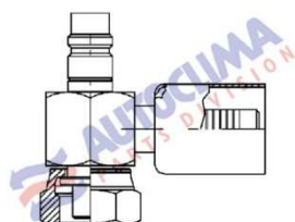
ŻEŃSKA - 90° - ROTOLOCK PORT R134a
