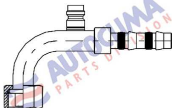
FRIGO - 90° - O.RING - ŻEŃSKA PORT R134a
